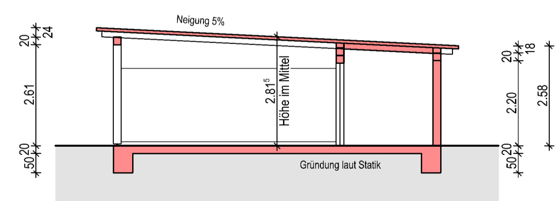
SCHNITT B-B
